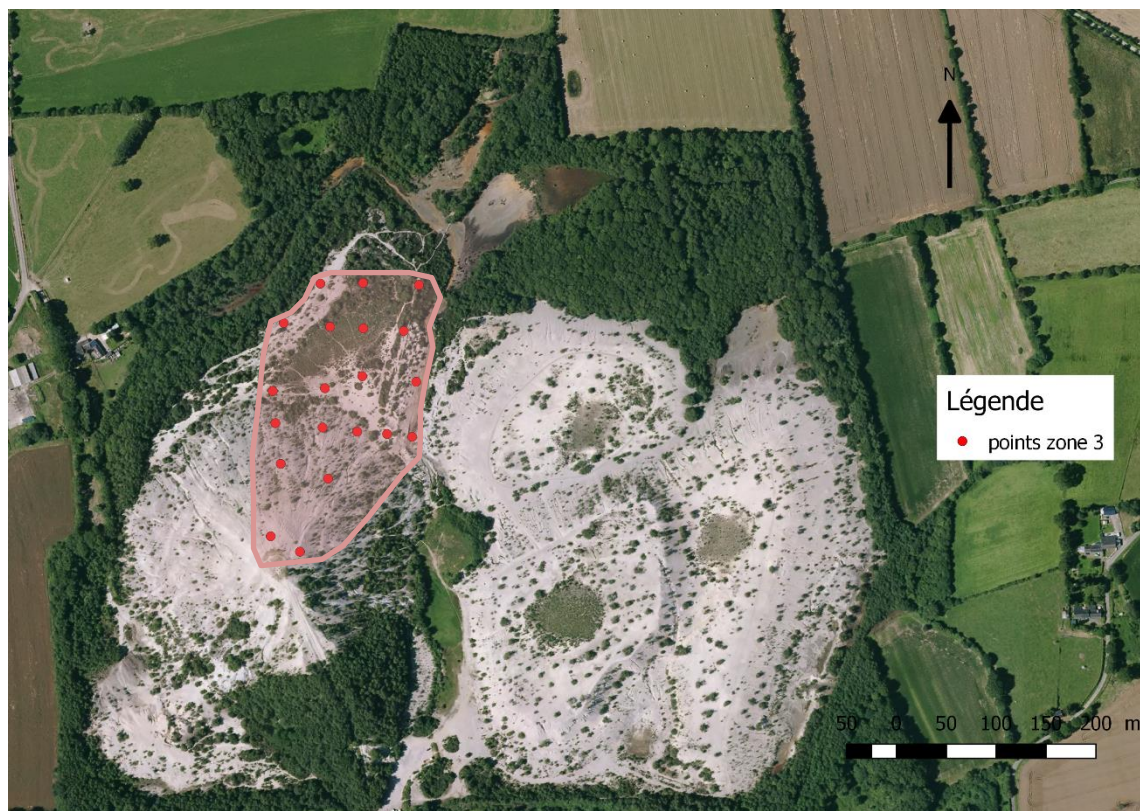
Illustration 75 - Délimitation de la zone 3 et localisation des mesures sélectionnées pour ce scénario.
