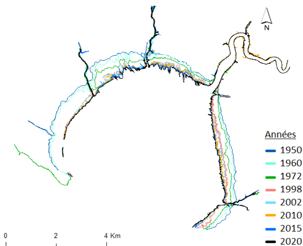
Figure 20 : Evolution de la limite du schorre de 1950 à 2020 (Olivier, 2021).
