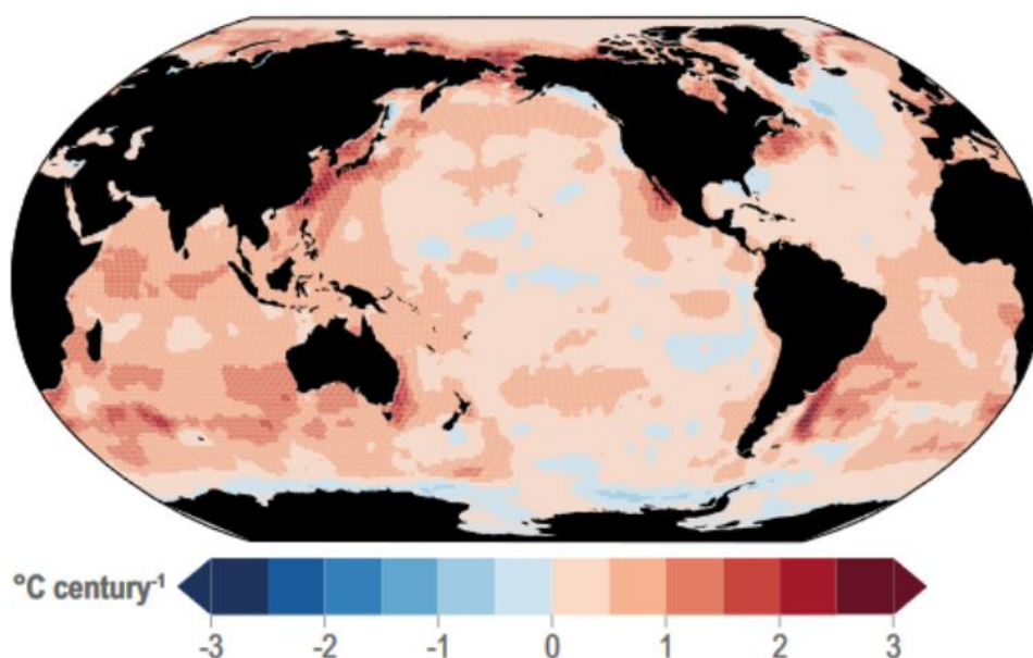
Figure 26 : Tendance de la température de la surface de la mer (degrés Celsius par siècle) entre 1925 et 2016 ((Hadley Centre Sea Ice and Sea Surface Temperature 1.1 (HadISST1)).
