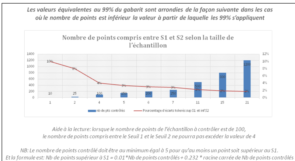
1 – gabarit 1 : Classe de précision A applicable aux réseaux neufs posés en fouille ouverte ou aux IC intrusives
