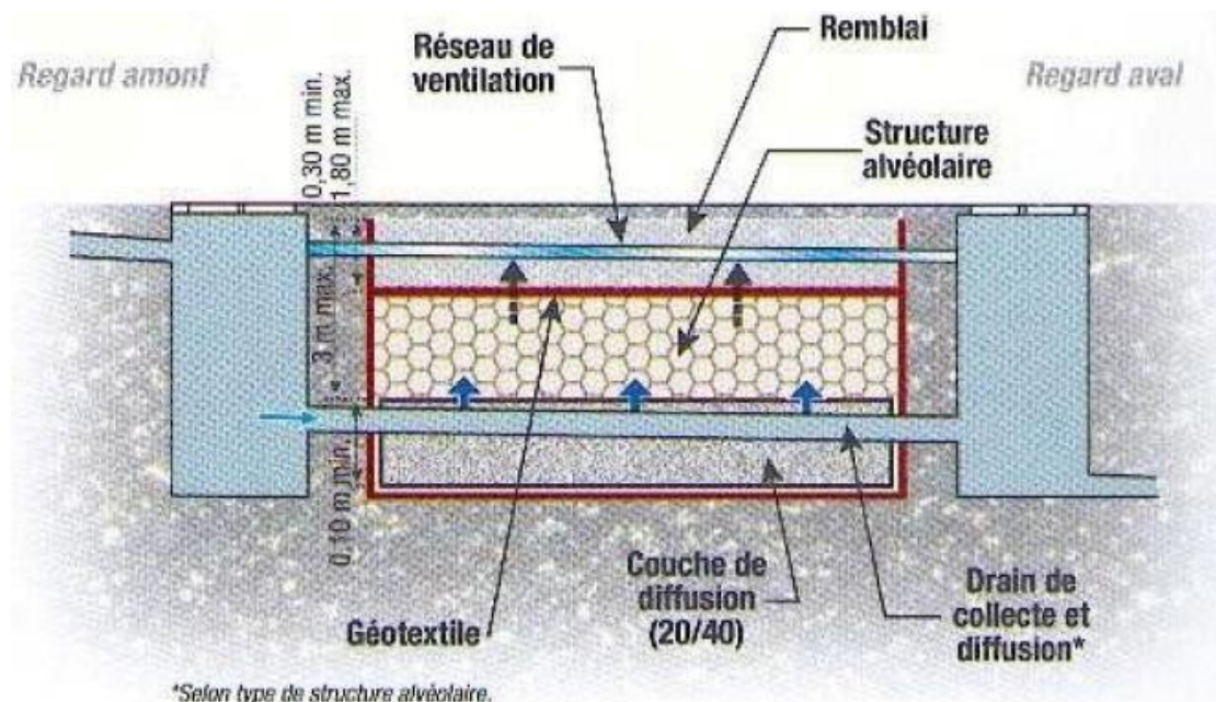
*Selon type de structure alvéolaire. Coupe type de SAUL (crédit image : ADOPTA, www.adopta.fr )
