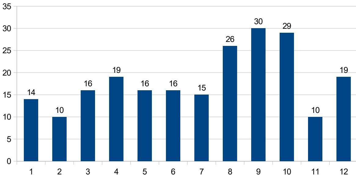
Nbre échéances avis MRAe /mois 2025
