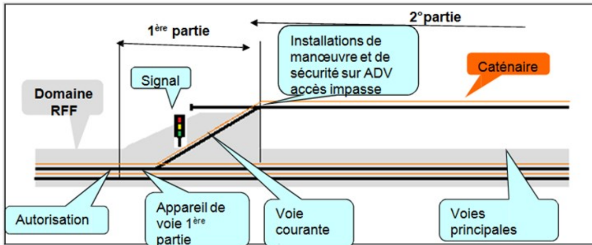
Illustration 154: Schéma de description d'une ITE
