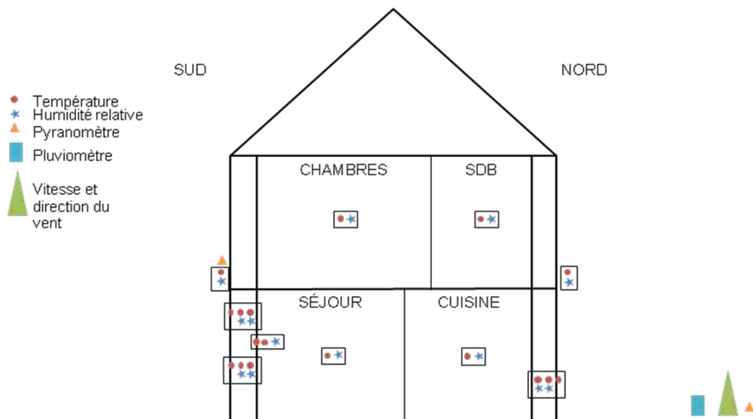
Figure 3-26 : Plan général de l'instrumentation approfondie
