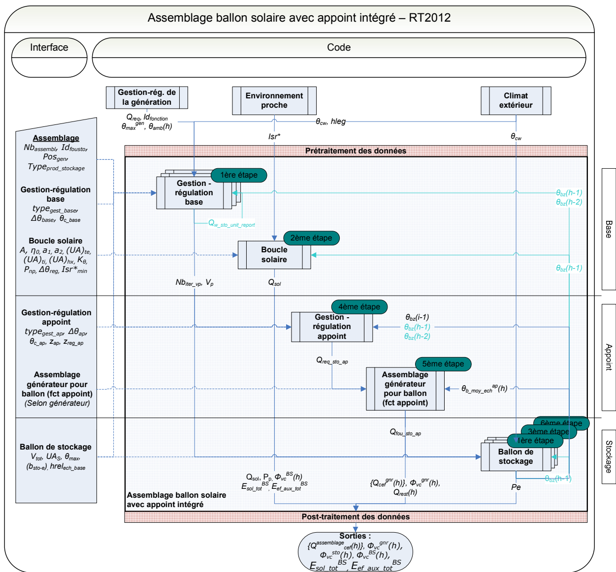
Figure 144 : Schéma d'assemblage du modèle de chauffe-eau solaire à appoint intégré
