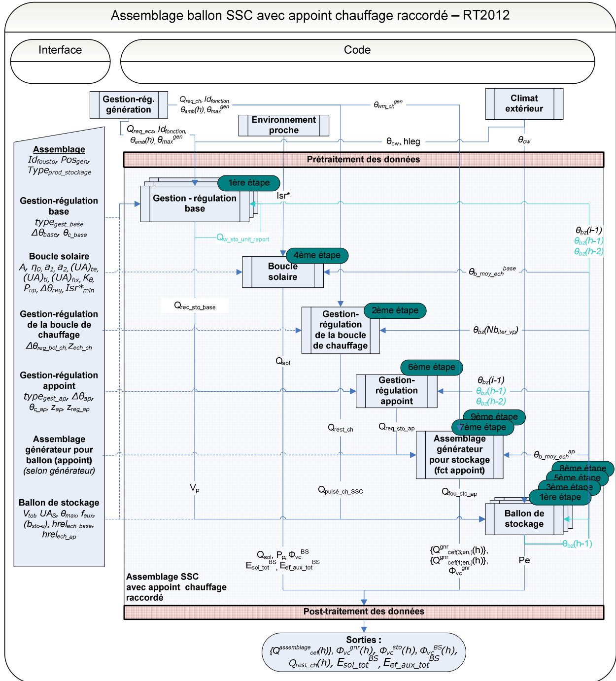
Figure 152 : schéma d'assemblage du modèle de système solaire combiné avec appoint pour le chauffage raccordé à l'assemblage
