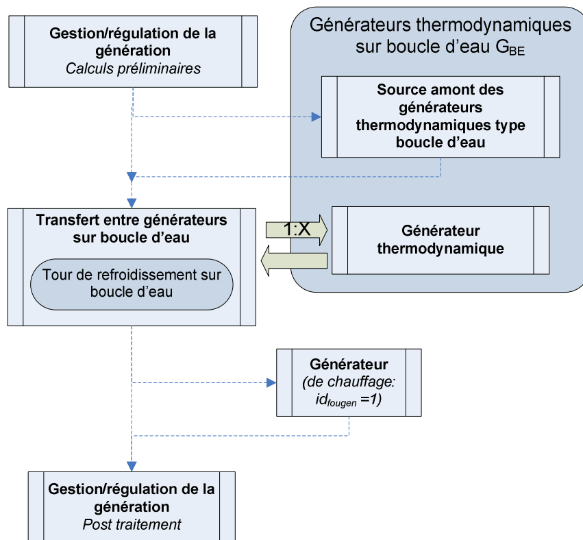
Figure 86 : Séquence d'appel des composants pour la modélisation d'une boucle d'eau
