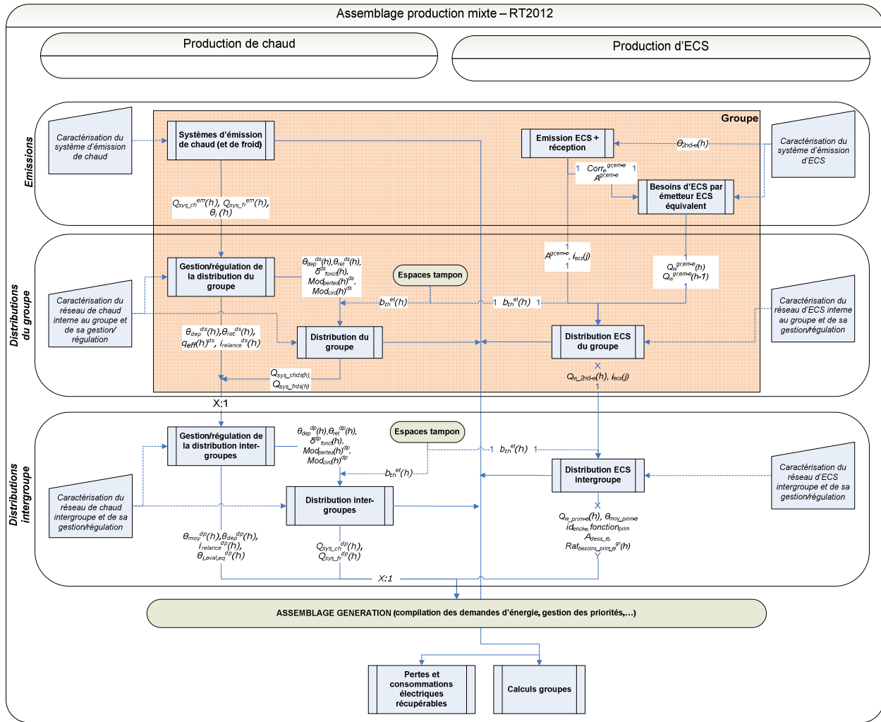
Figure 139 : Schéma d'assemblage de la production mixte ECS/chauffage
