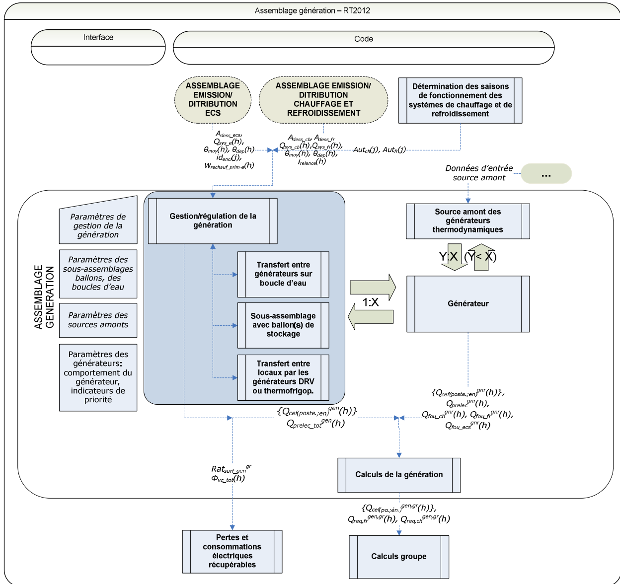
Figure 85 : Assemblage de la génération
