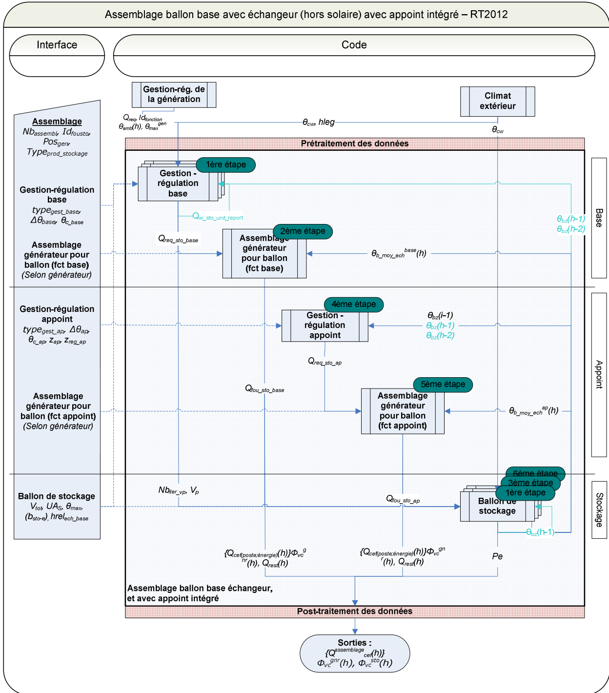
Figure 145 : Schéma d'assemblage du modèle de chauffe-eau base avec échangeur et à appoint intégré
