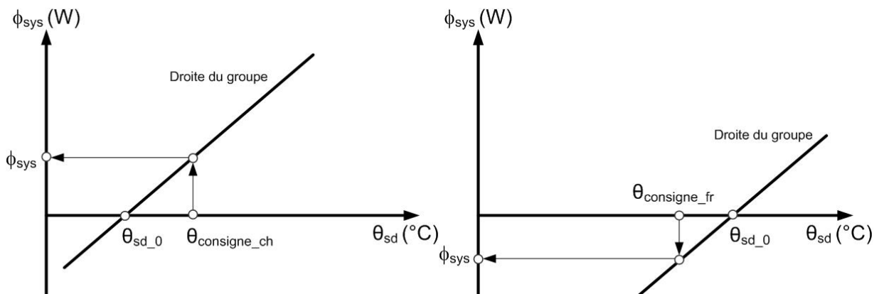
Figure 78 : Intersection avec la droite du groupe
