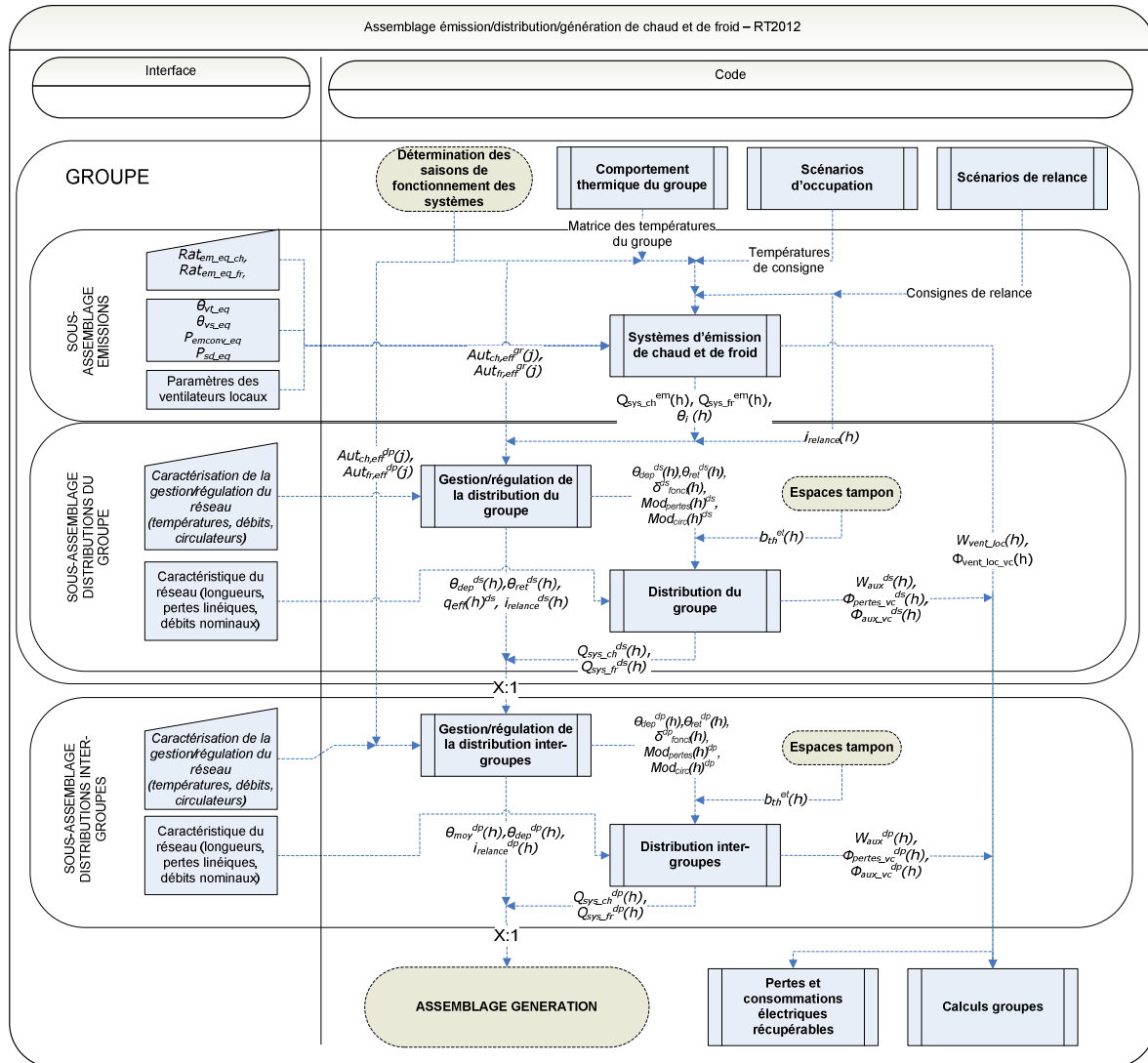
Figure 82: Assemblage des composants des systèmes de chauffage et de refroidissement
