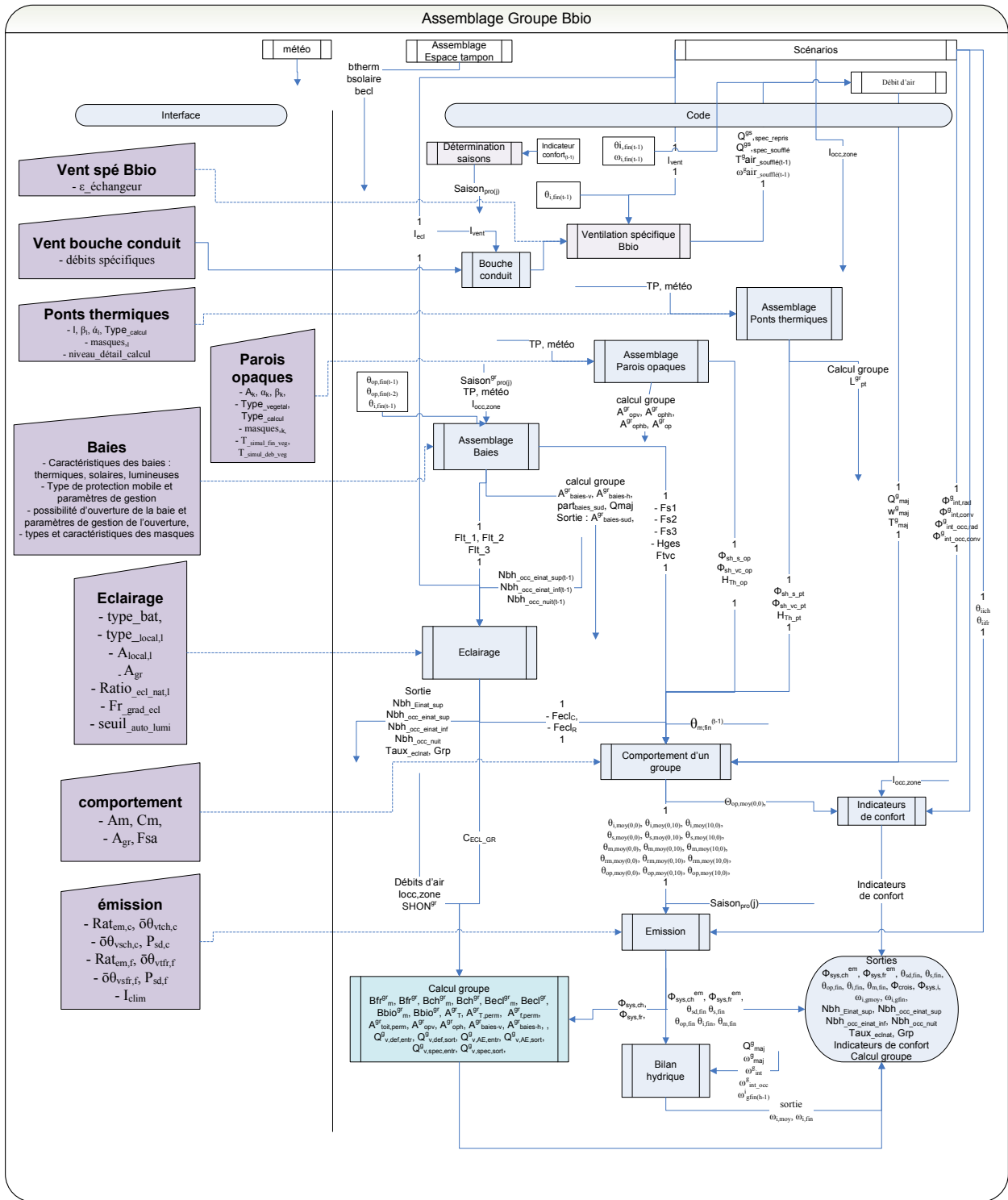
Figure 16 : Assemblage des composants d'un groupe pour le calcul de Bbio
