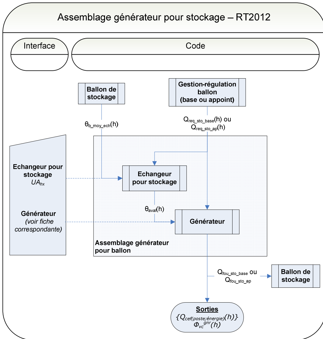
Figure 142 : schéma d'assemblage du modèle de générateur pour stockage
