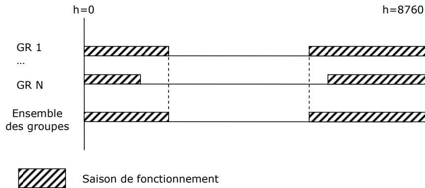
Figure 79: illustration de la procédure de détermination des saisons au niveau de la génération
