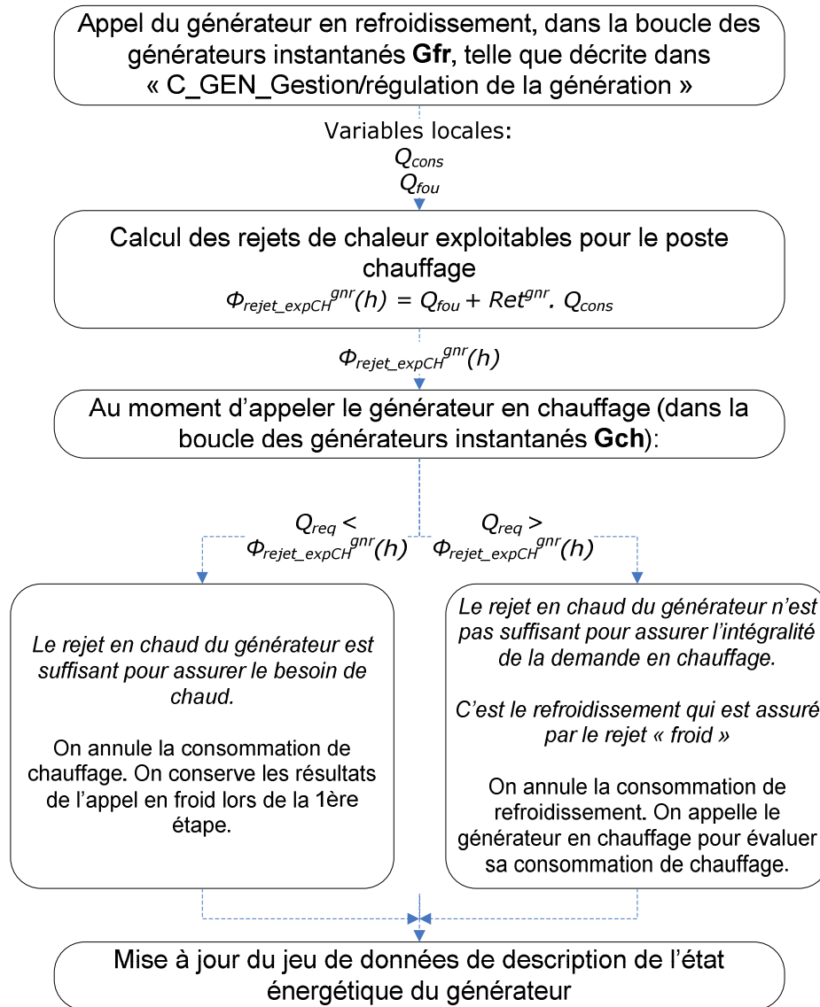
Figure 87: Description du processus de calcul horaire des transferts d'énergie par les générateurs DRV et thermofrigopompes
