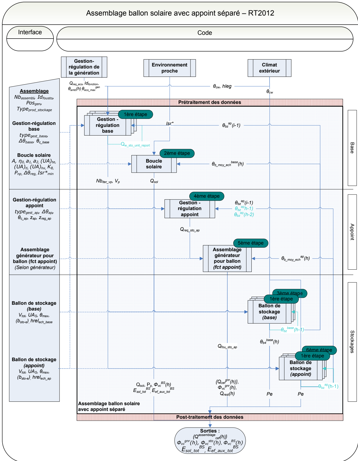
Figure 146 : Schéma d'assemblage du modèle de chauffe-eau solaire à appoint ballon séparé
