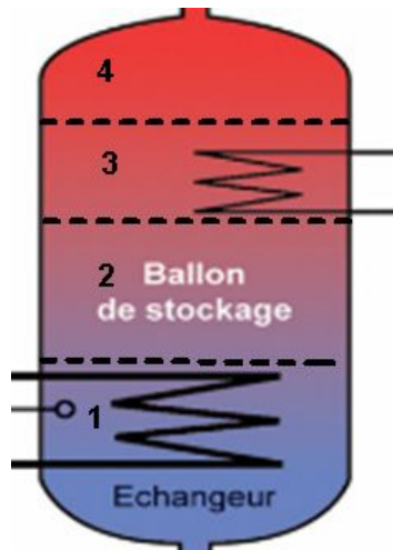
Figure 141 : schéma du ballon à quatre zones
