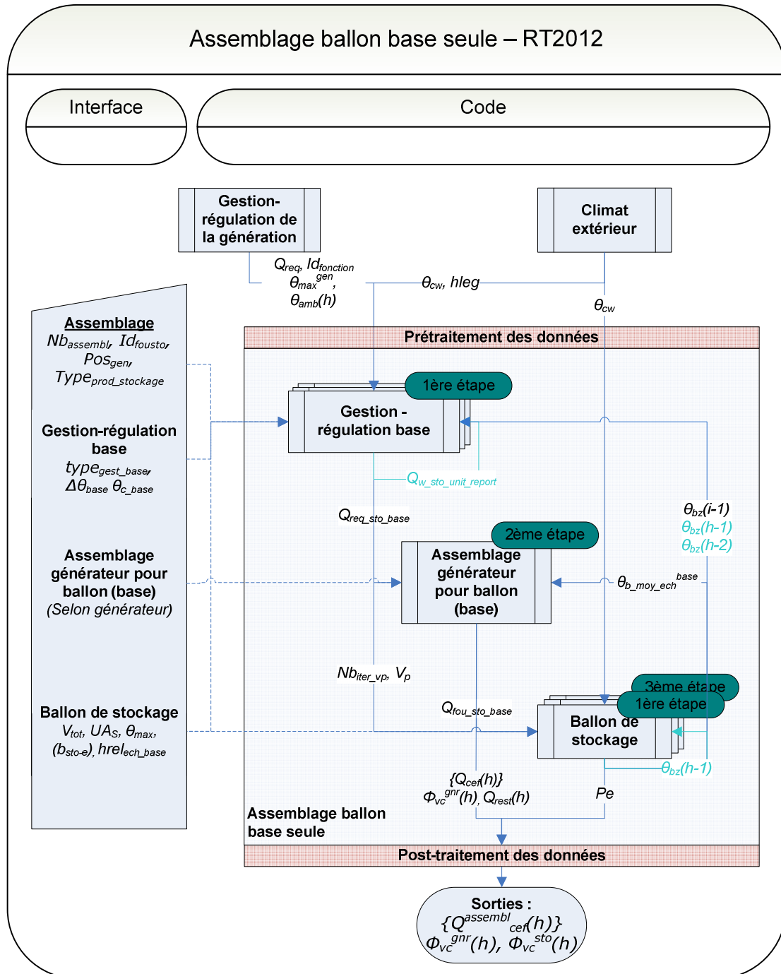
Figure 143 : Schéma d'assemblage du modèle de ballon base seule
