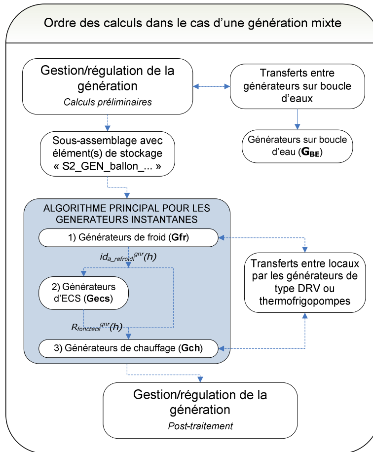
Figure 88: ordre des calculs dans la génération
