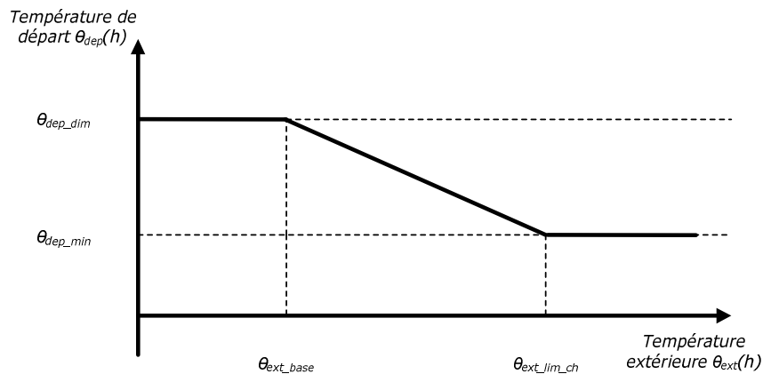
Figure 84 : Evolution de la température de départ en fonction de la température extérieure
