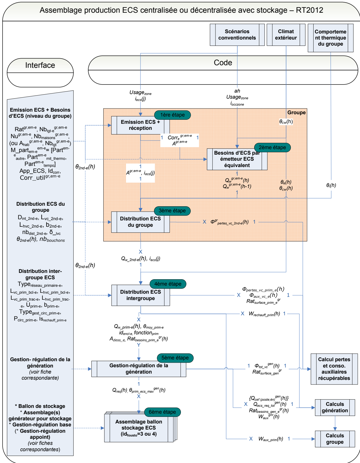
Figure 138 : Schéma d'assemblage de la production d'ECS avec stockage
