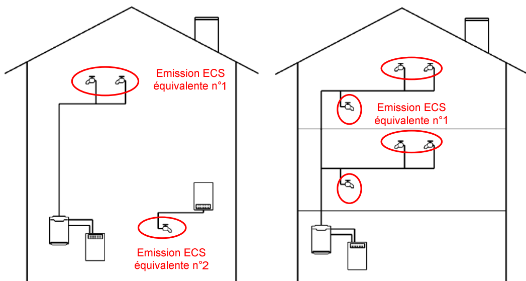
Figure 140 : Exemples de découpage en émetteurs_ECS avec respectivement 2 ou 1 génération(s) (schémas issus de la NF EN 15316-3-2)
