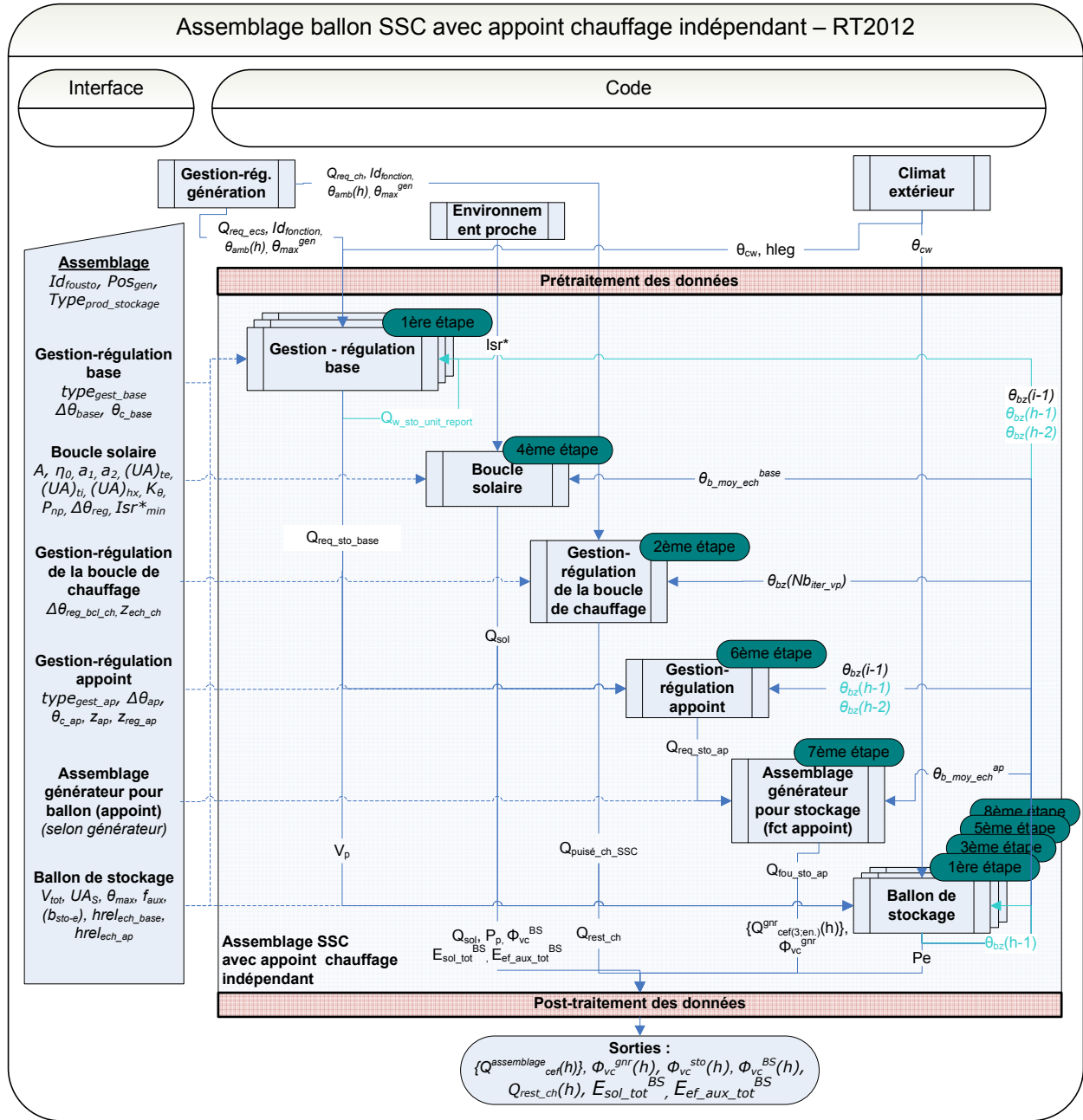
Figure 151 : schéma d'assemblage du modèle de système solaire combiné avec appoint indépendant pour le chauffage
