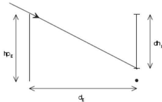
Figure 3 : Masque lointain défini par un plan vertical
