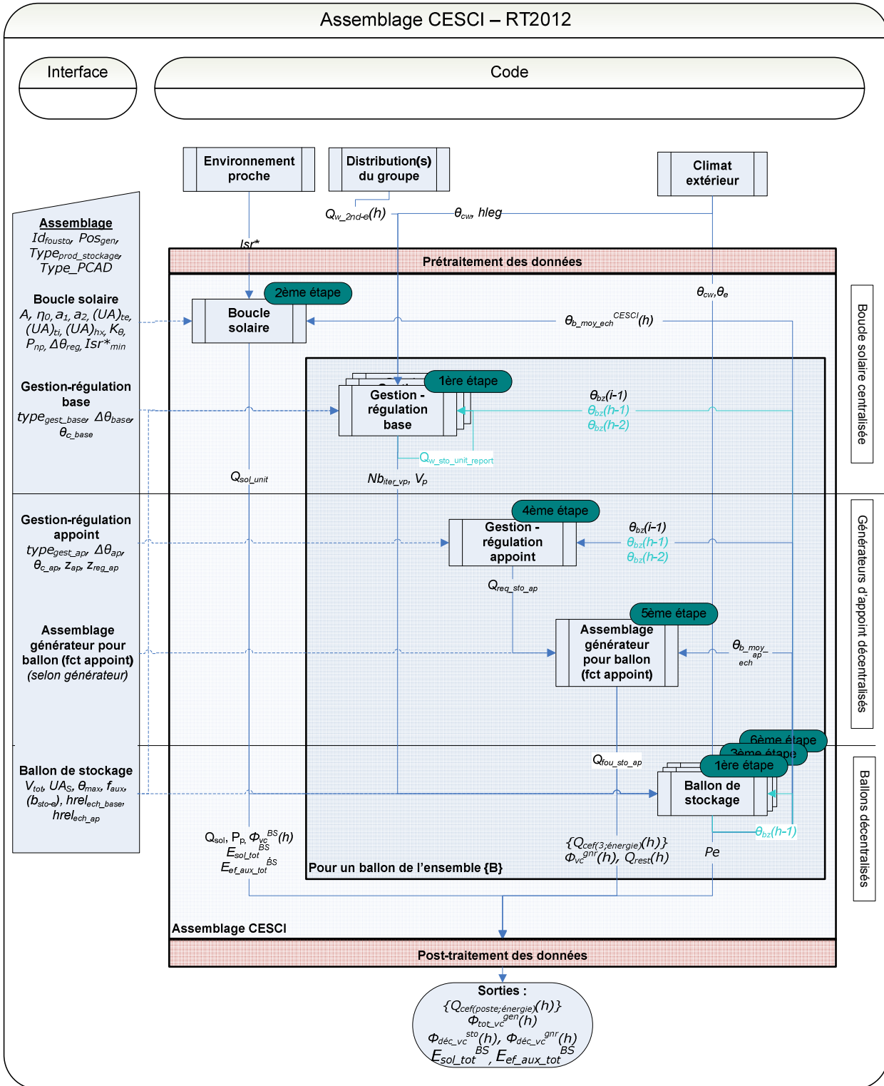
Figure 150 : Schéma d'assemblage du modèle de CESCOI
