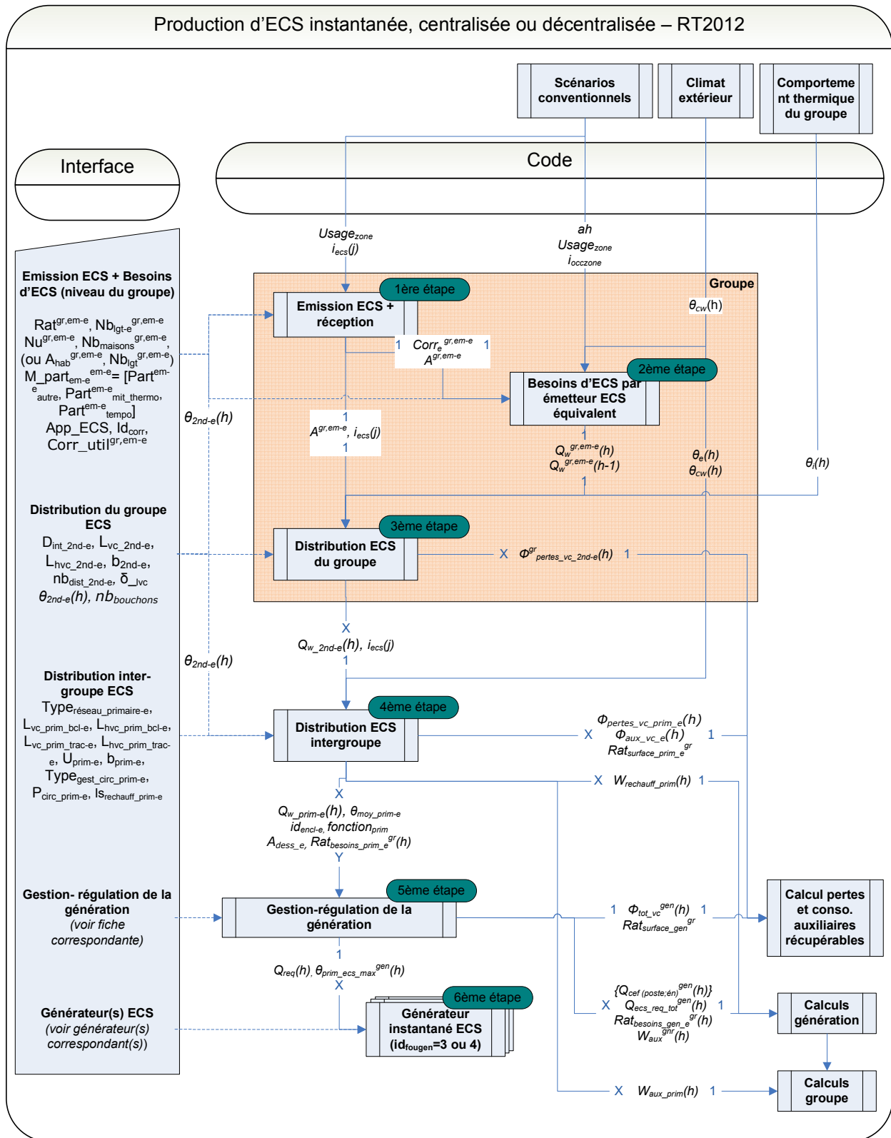
Figure 137 : Schéma d'assemblage de la production instantanée d'ECS
