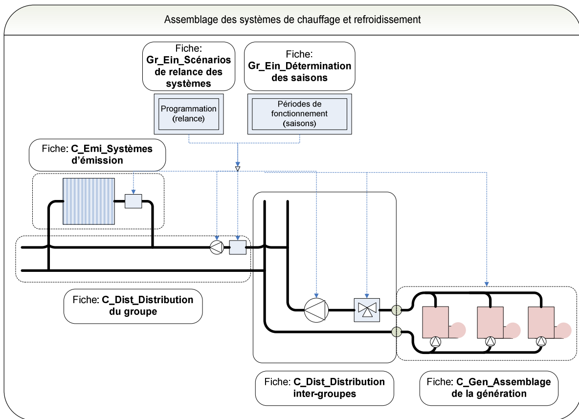
Figure 81: Assemblages des systèmes de chauffage et de refroidissement
