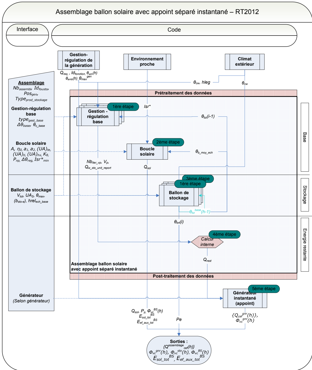
Figure 148 : Schéma d'assemblage du modèle de chauffe-eau solaire à appoint séparé instantané
