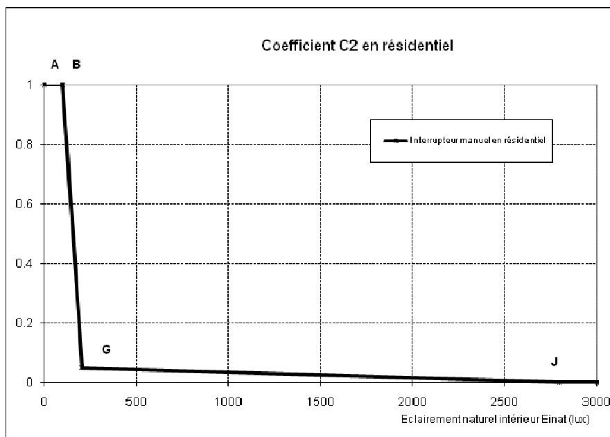
Figure 76 : Courbe donnant les valeurs de C2 selon l’éclairement naturel intérieur en résidentiel
