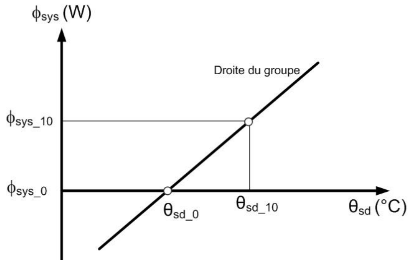
Figure 77 : Droite de comportement thermique d'un groupe
