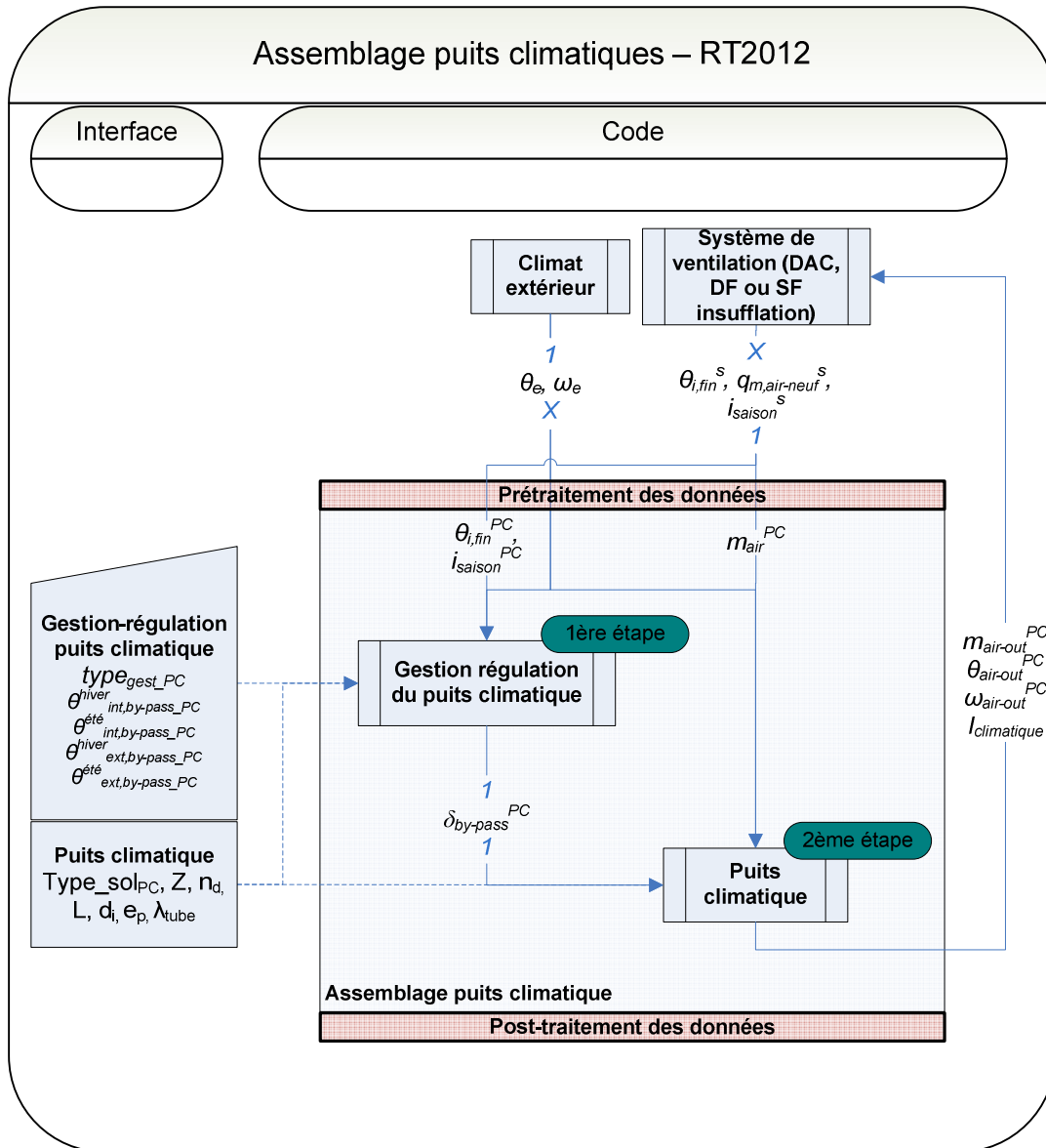
Figure 73 : Schéma d'assemblage du modèle de puits climatique
