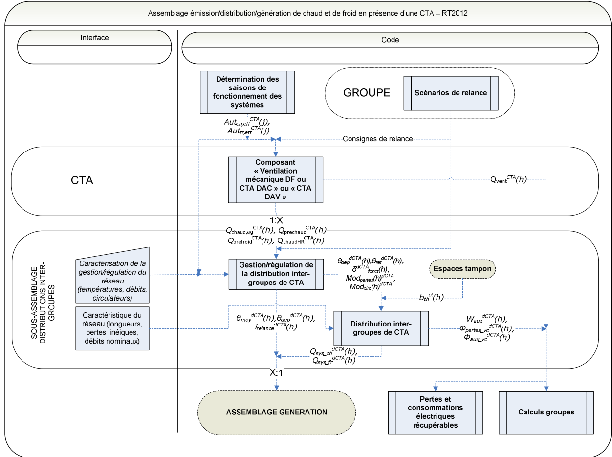
Figure 83 : Assemblage des composants des systèmes associés à une CTA
