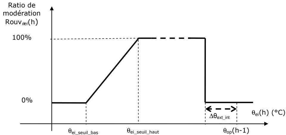
Figure 18: ratio de modération de l'ouverture en fonction de la température extérieure
