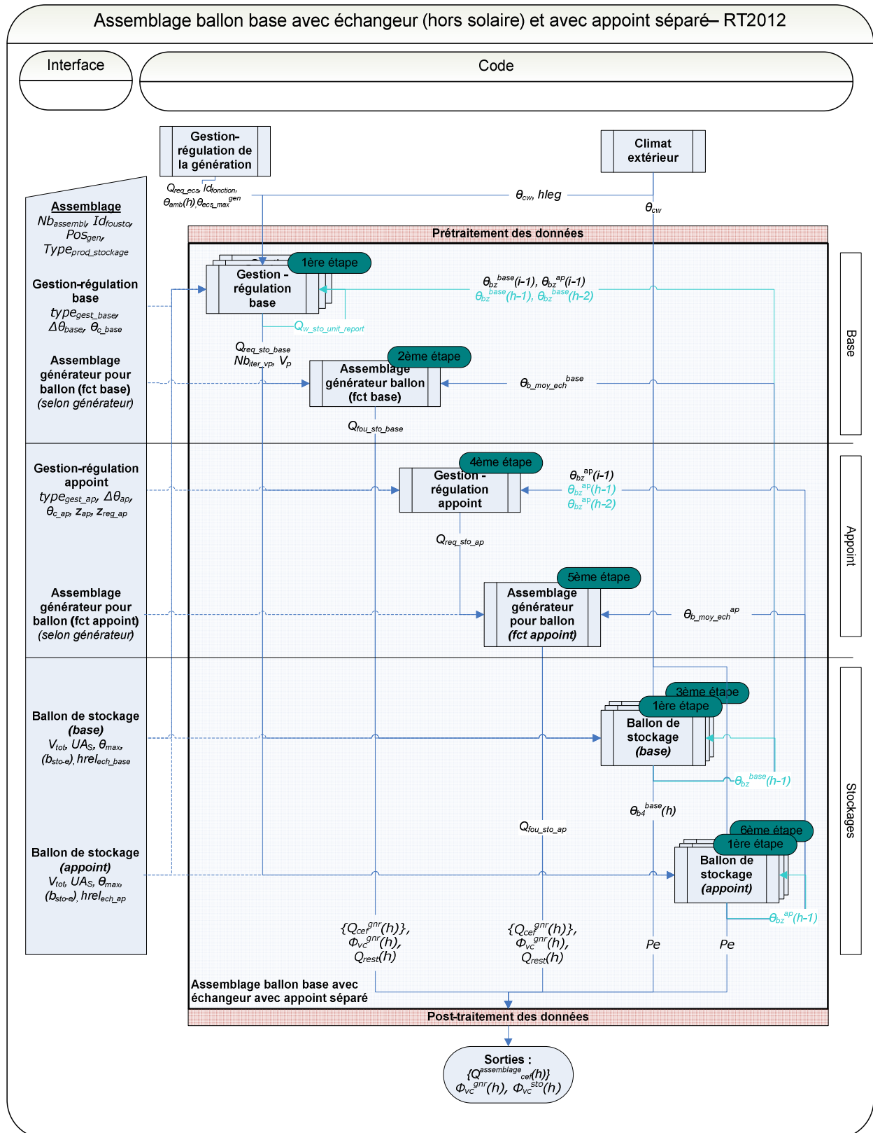
Figure 147 : Schéma d'assemblage du modèle du ballon base avec échangeur et avec appoint ballon séparé
