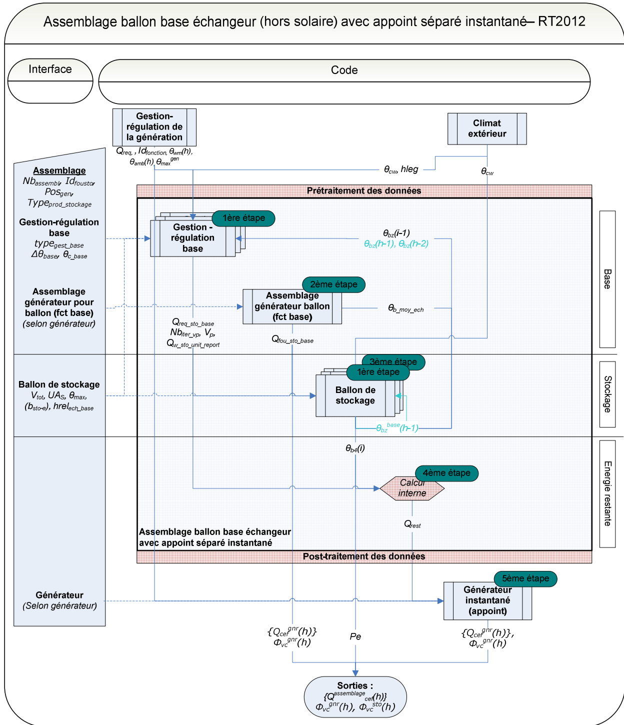
Figure 149 : Schéma d'assemblage du modèle de chauffe-eau avec base échangeur et à appoint séparé instantané
