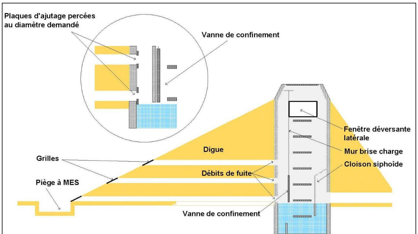
Figure 16 : Ouvrage de régulation et de traitement en sortie de bassin tampon (cas d'un lotissement)
