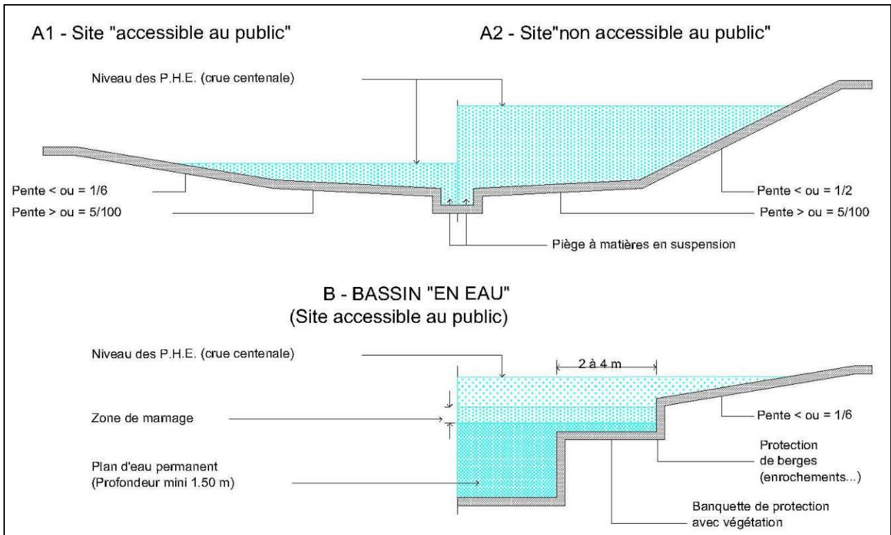
Figure 15 : Profil en travers type de bassins tampon
