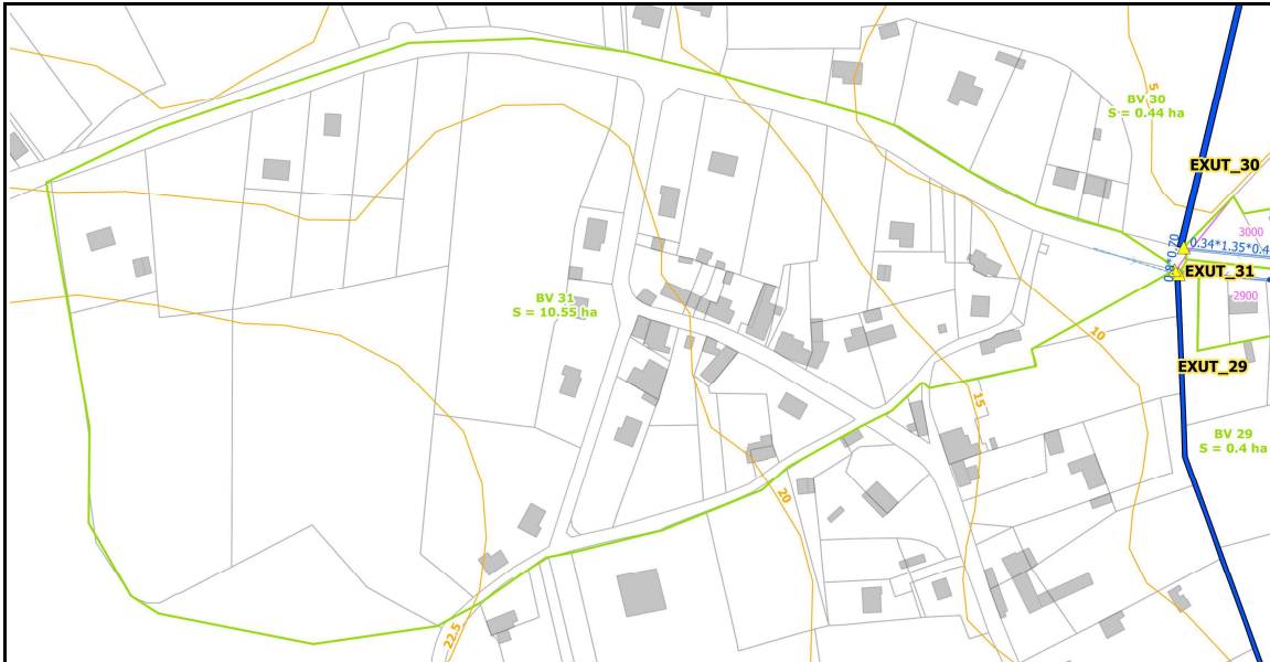
Figure 11 : Réseau pluvial et bassins versants, exutoire 31
