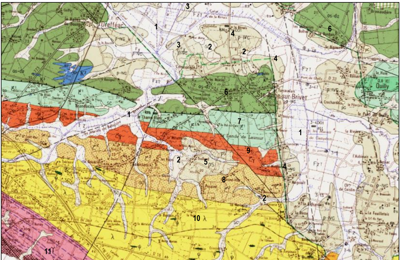
Figure 6 : Extrait de la carte géologique de SAINTE-ANNE-SUR-BRIVET (carte géologique 1/50 000_feuille de SAVENAY source BRGM)
