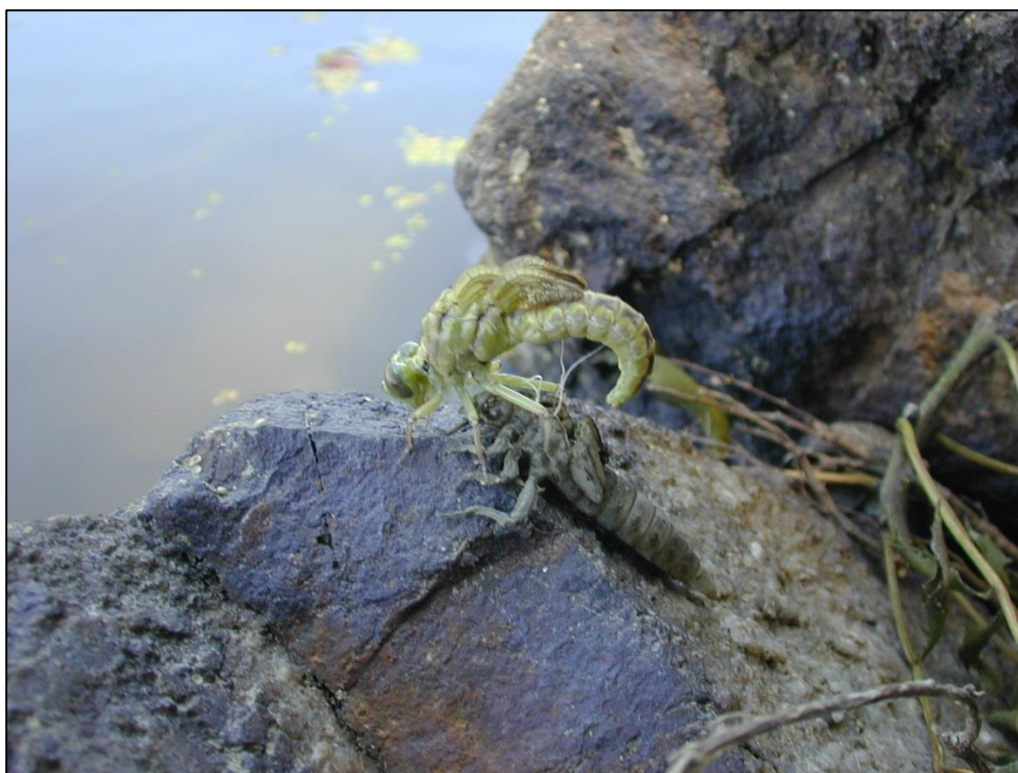
Imago de Gomphus flavipes venant d'émerger, inapte au vol, situé juste au-dessus de l'eau ; on imagine aisément l'impact que pourrait avoir le batillage sur de tels individus.
