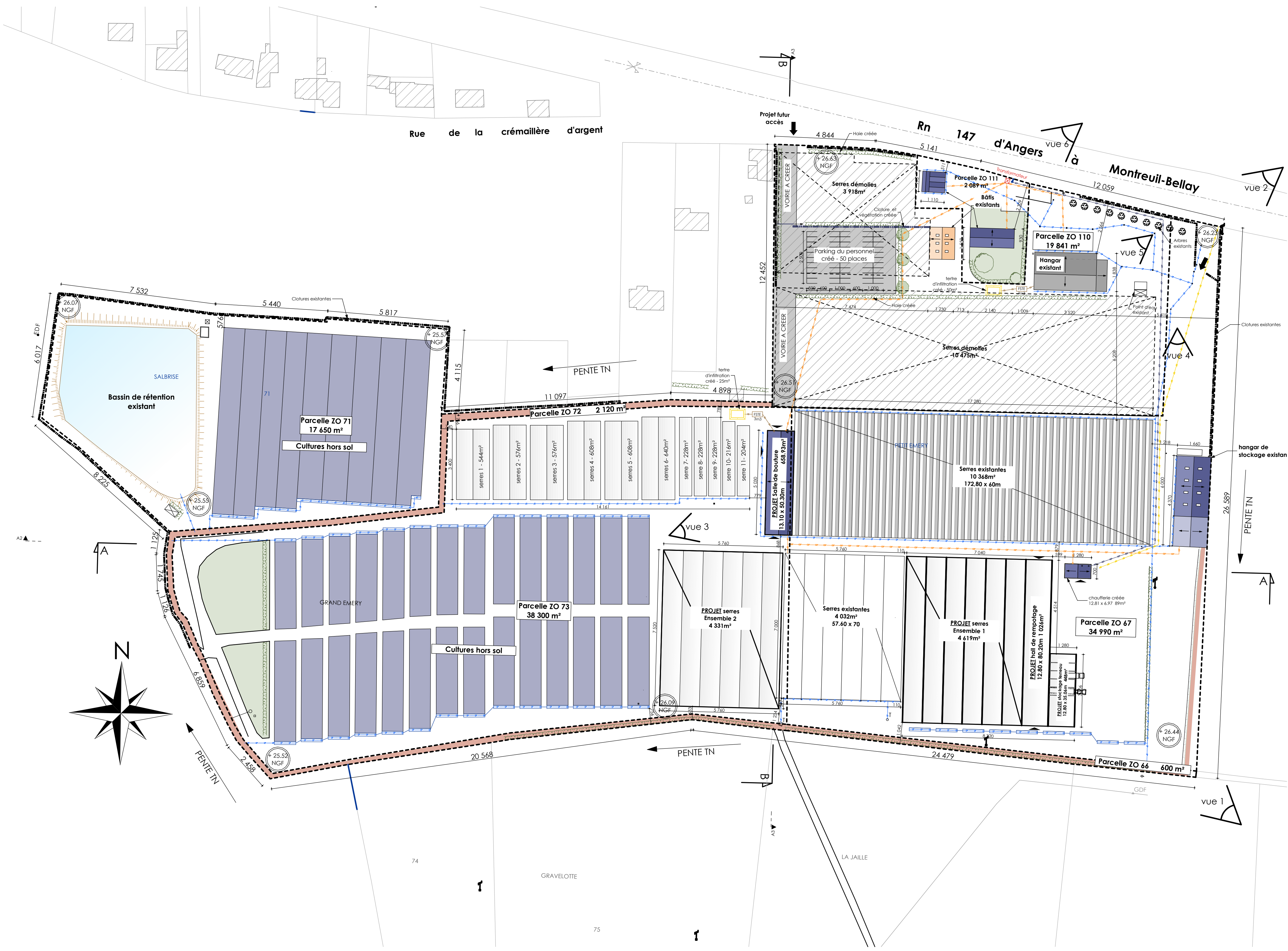
PC 2 - PLAN DE MASSE PROJET - 1/1000°
